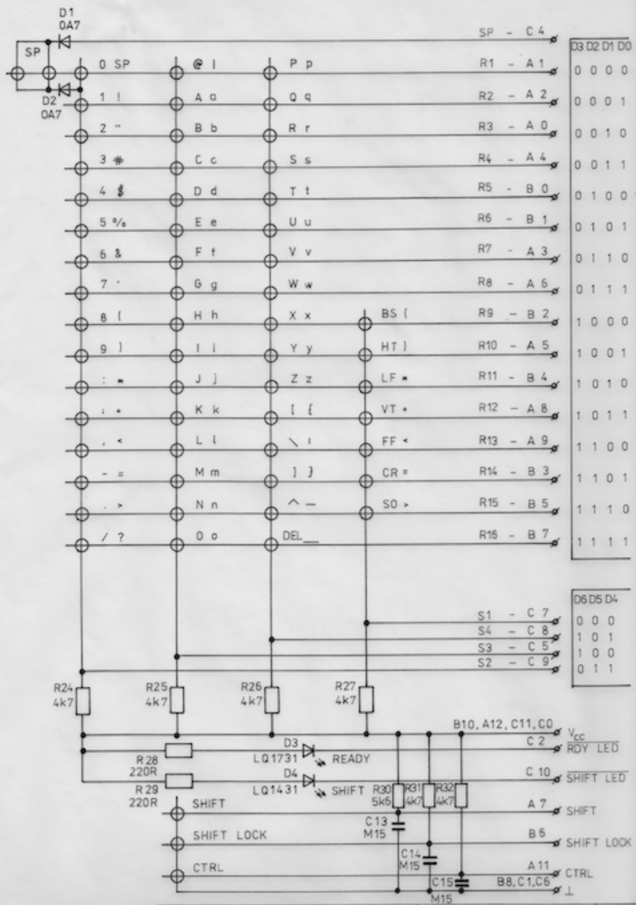
15 | PLAN 80A - KONTAKTNÍ KLÁVESNICE - MATICE KLÁVES
